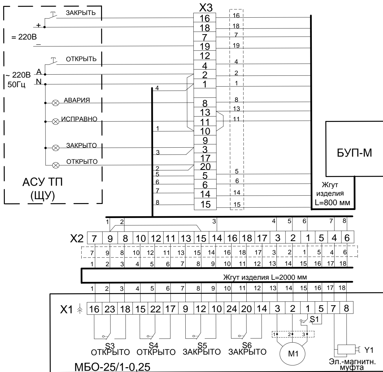
Схема электрическая подключений электромеханизма МБО-25/1-0,25 с блоком управления БУП-М при наличии на объекте источника постоянного напряжения 220В
