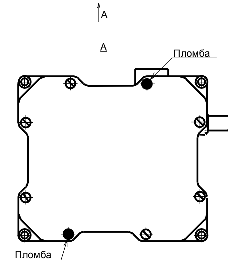
Габаритные и присоединительные размеры, места пломбировки блока БУП М3О-125
