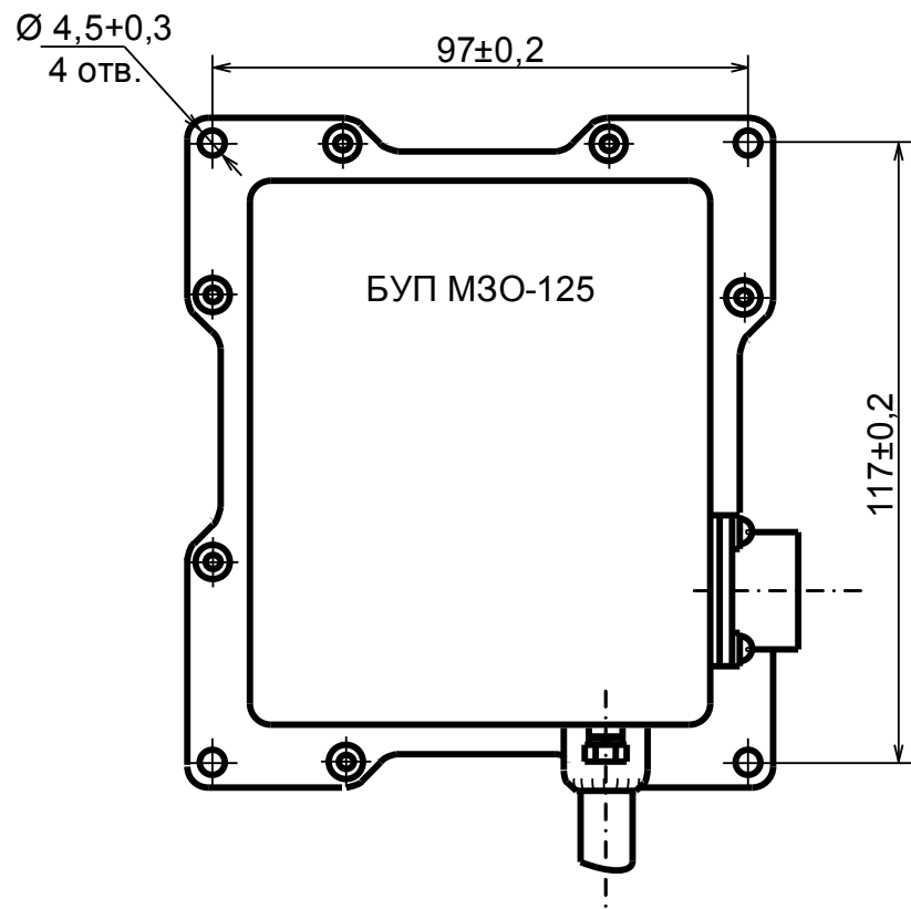
Габаритные и присоединительные размеры, места пломбировки блока БУП М3О-125
